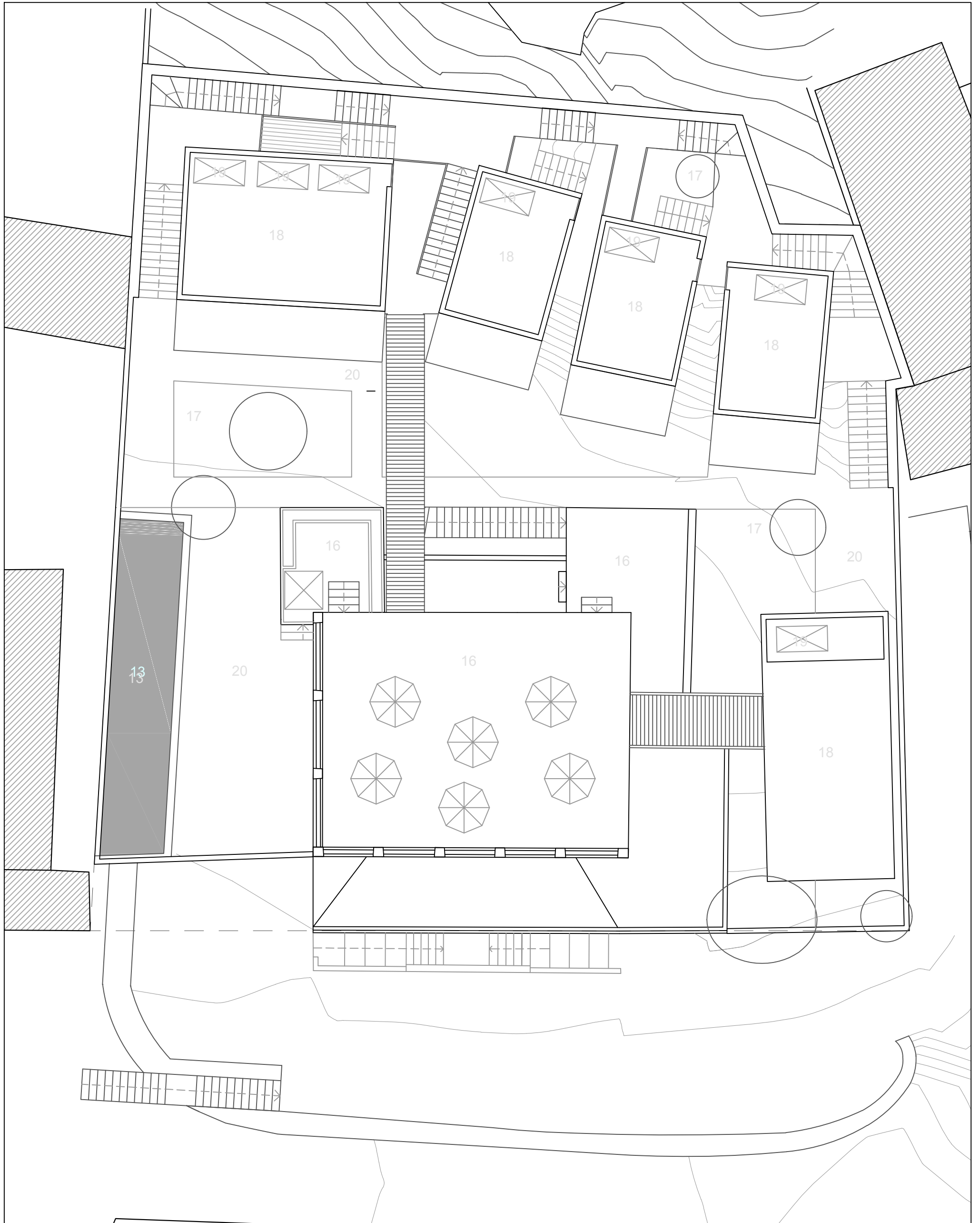
PLANTA COBERTURA - GERAL escala 1 : 200
